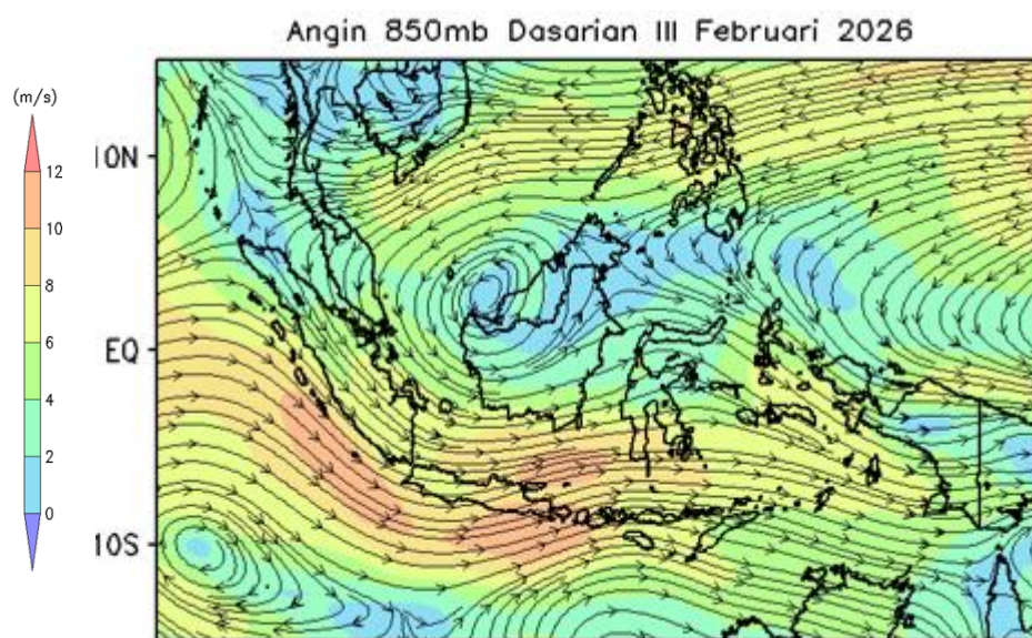
Gambar 7. Analisis Streamline Angin Februari 2026
