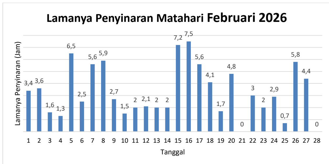
Gambar 13. Grafik Lama Penyinaran Matahari Bulan Februari 2026
