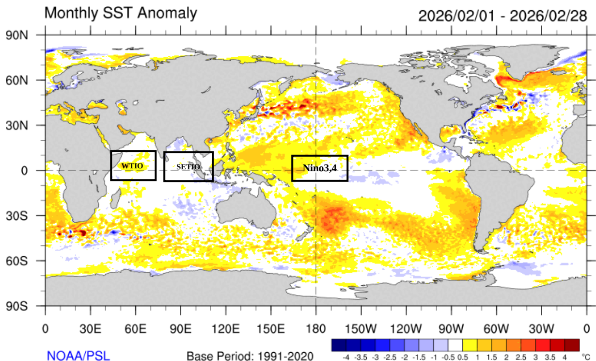
Gambar 2. Anomali Suhu Muka Laut Bulan Februari 2026
