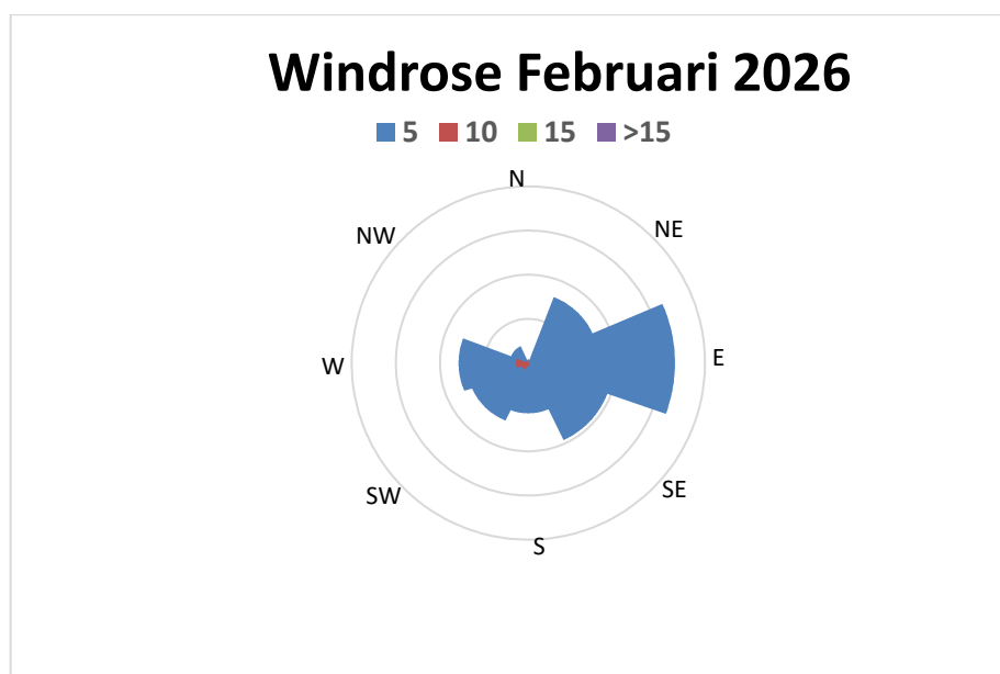
Gambar 10. Wind Rose Bulan Februari 2026
