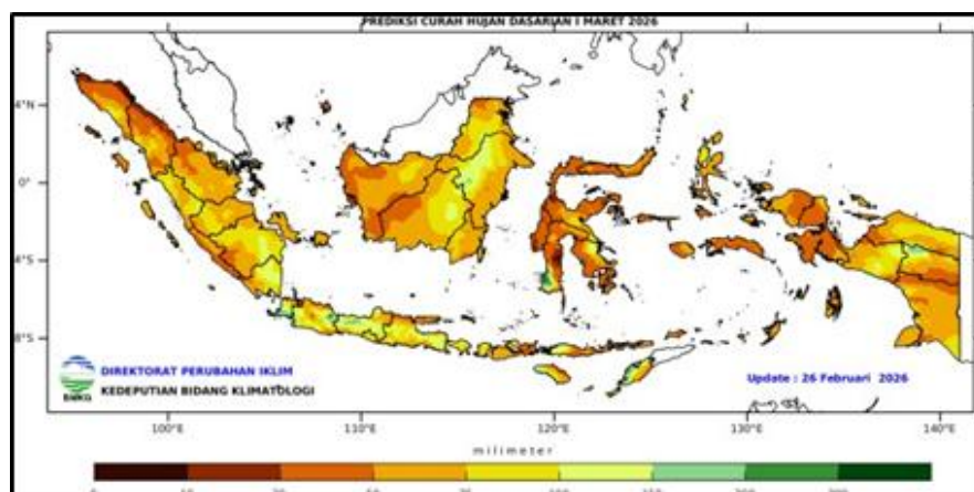
Gambar 16. Prediksi Curah Hujan Dasarian 1 Maret 2026
