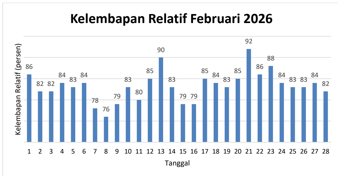
Gambar 12. Grafik kelembapan udara relatif bulan Februari 2026
