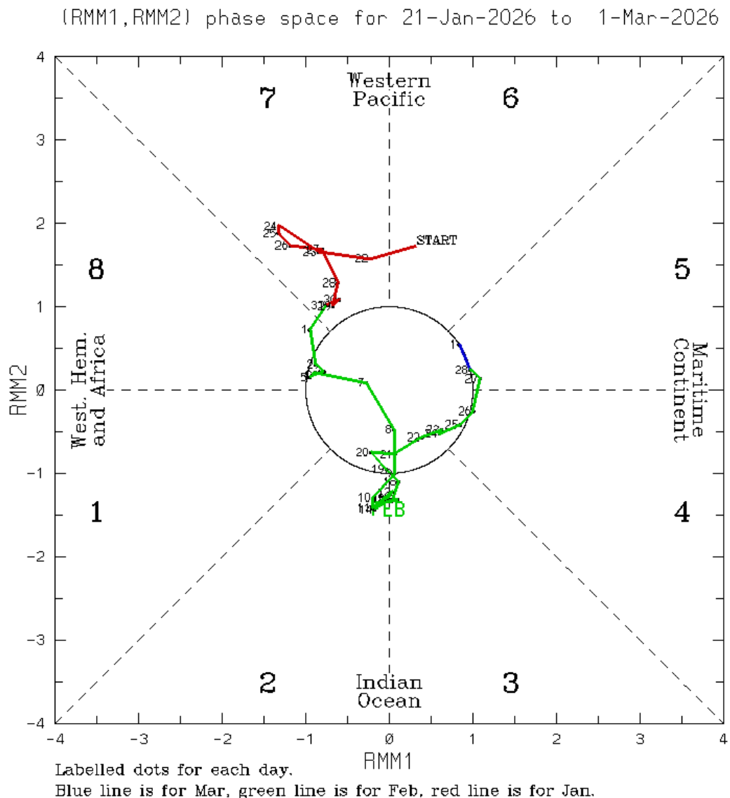
Gambar 6. Fase MJO Bulan Februari 2026
