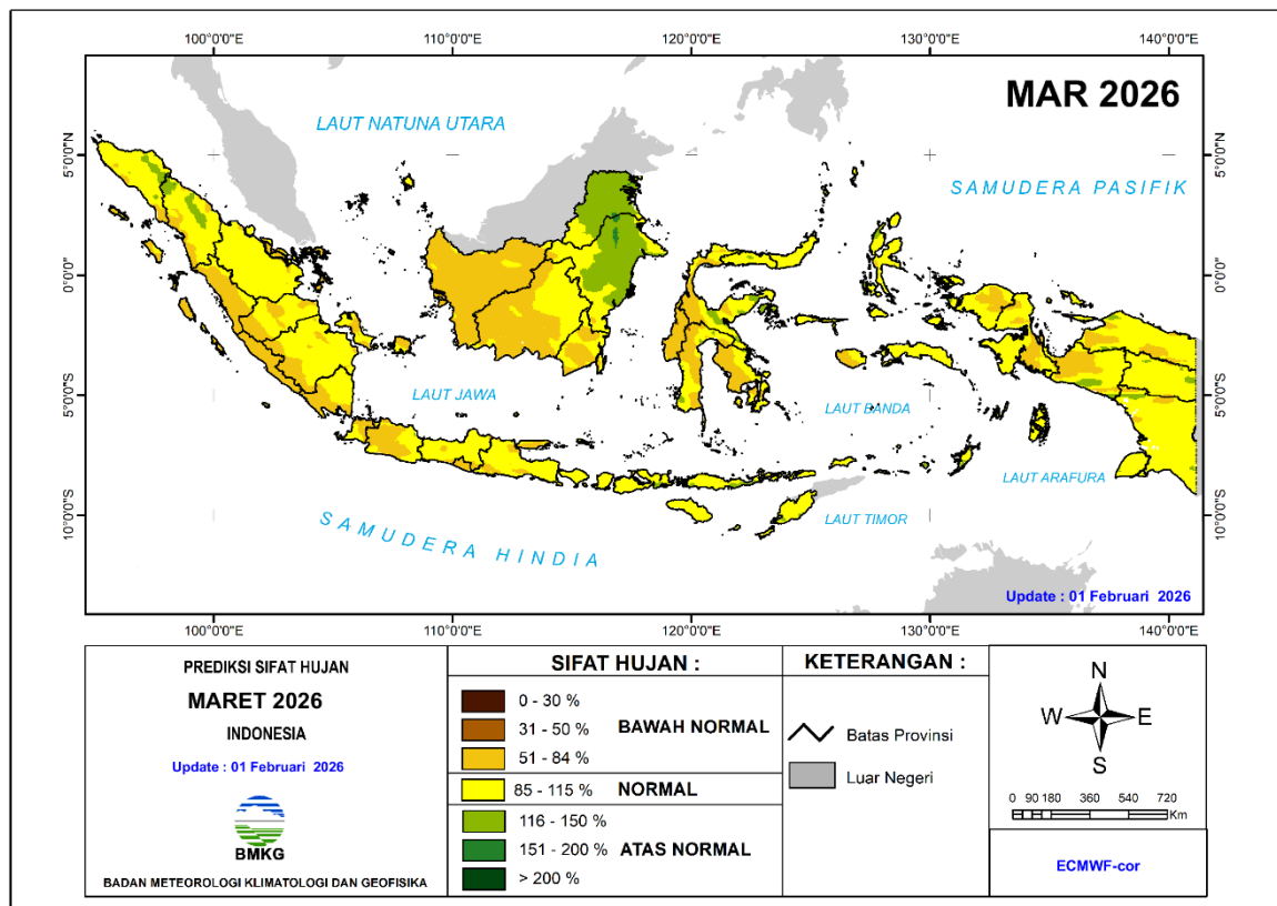
Gambar 15. Prediksi Sifat Hujan Bulan Maret 2026
