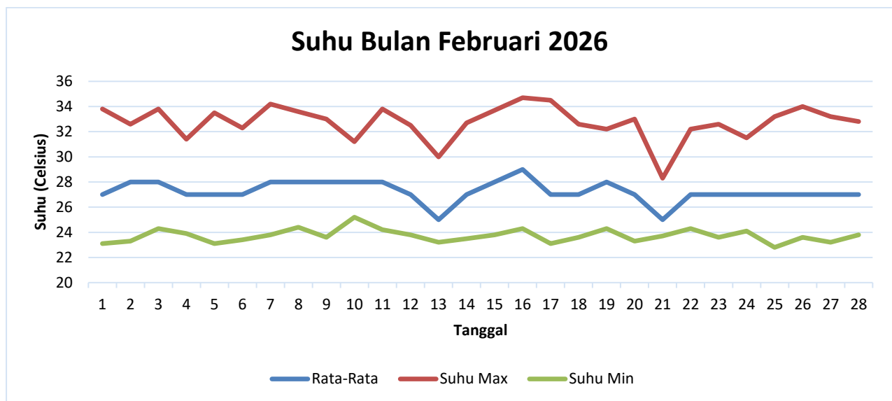
Gambar 11. Grafik Suhu Udara Bulan Februari 2026
