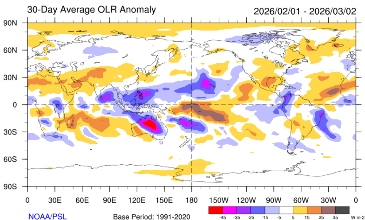
Gambar 4. OLR Anomali Bulan Februari 2026
