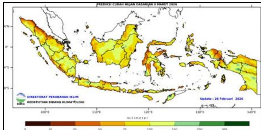
Gambar 17. Prediksi Curah Hujan Dasarian 2 Maret 2026
