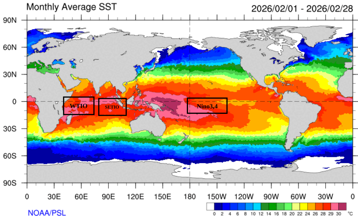
Gambar 1. Rata – rata Suhu Muka Laut Bulan Februari 2026
