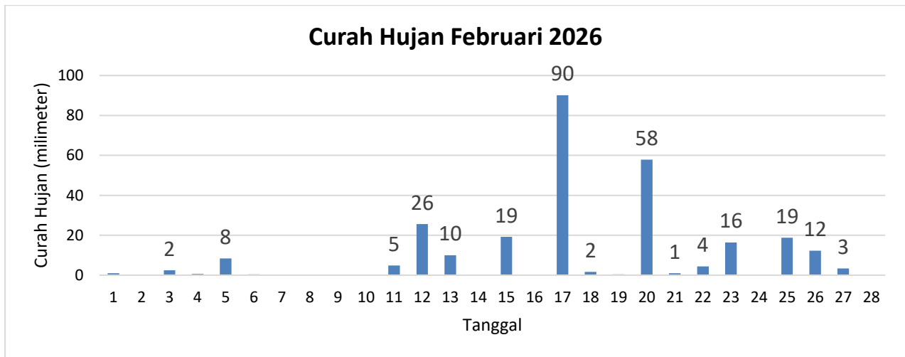
Gambar 9. Grafik Curah Hujan Bulan Februari 2026
